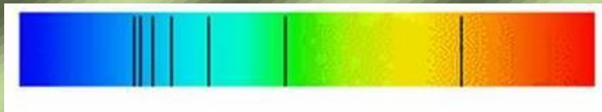
Hot star
